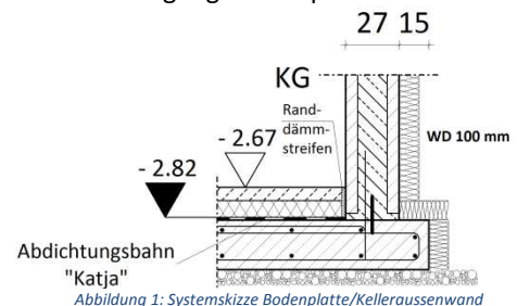
Abbildung 1: Systemskizze Bodenplatte/Kelleraußenwand
